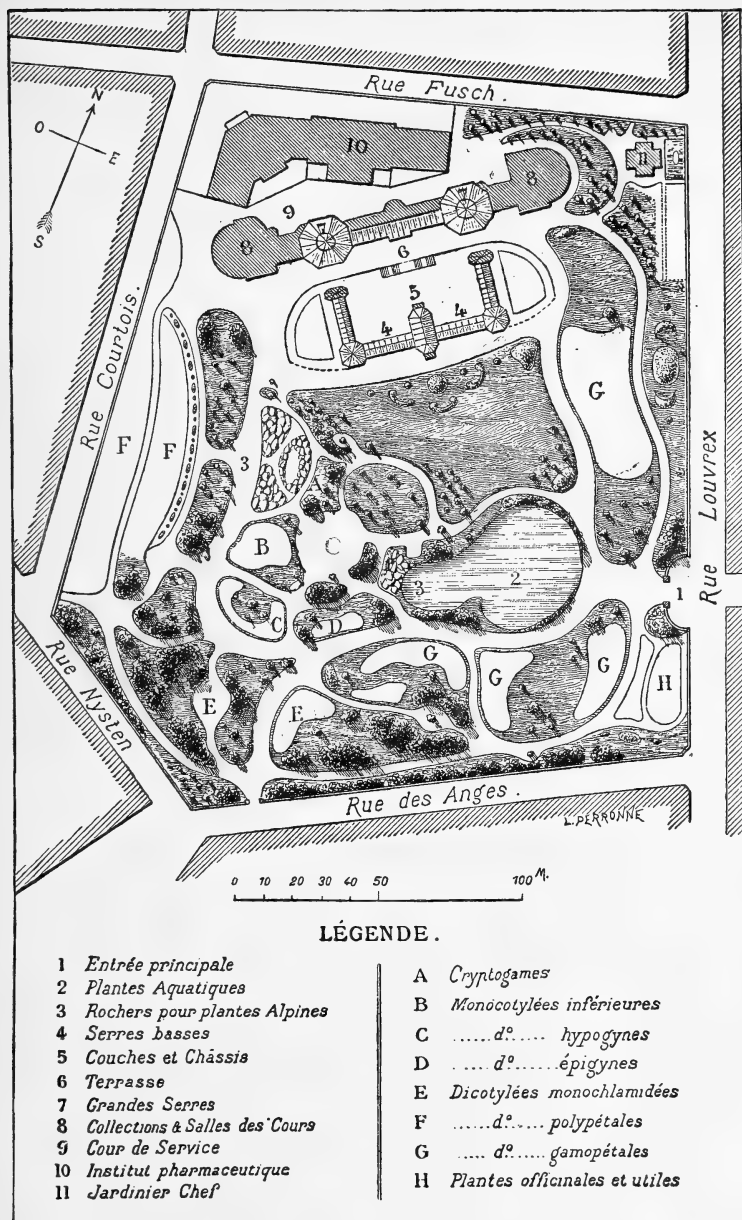
PLAN GÉNÉRAL.
